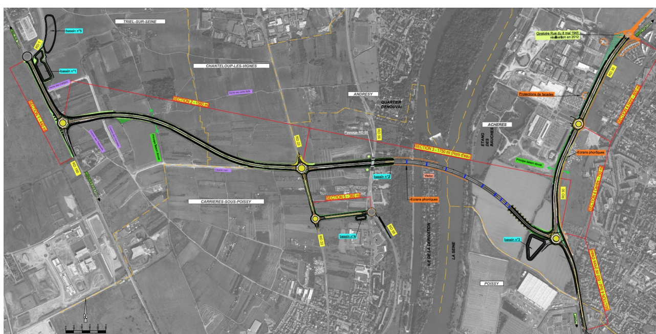
Figure 2: Projet de liaison entre la RD 190 et la RD 30, plan général des travaux - source : arrêté de DUP, 2013
